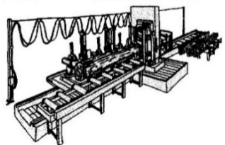
自動送材車付帯のこ盤
